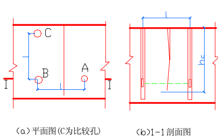
图 5.4.3 钻孔测裂缝深度示意图
