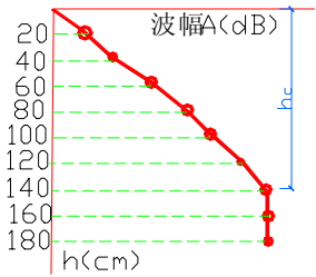
图 5.4.6 h-A 坐标图
