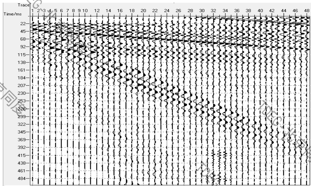
图 4.1c 7.5 万焦尔激震记录
