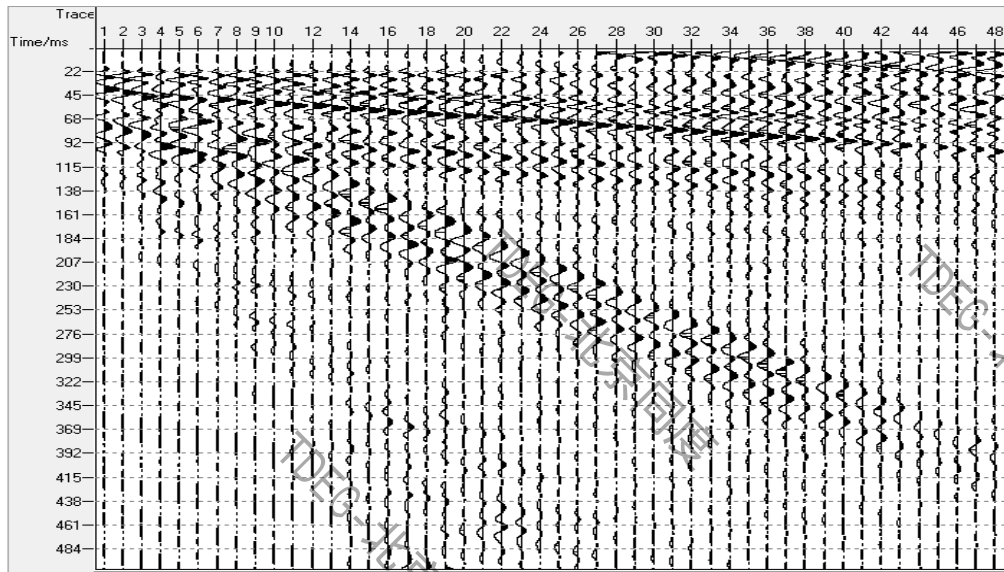
图 4.1b 5.0 万焦尔激震记录
