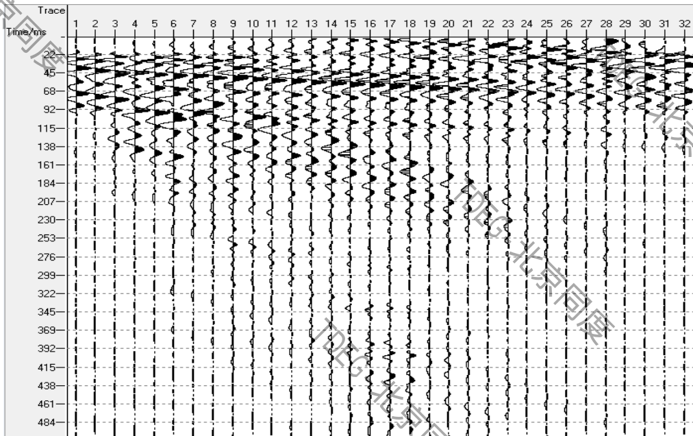
图 4.1a 2.5 万焦耳激震记录
